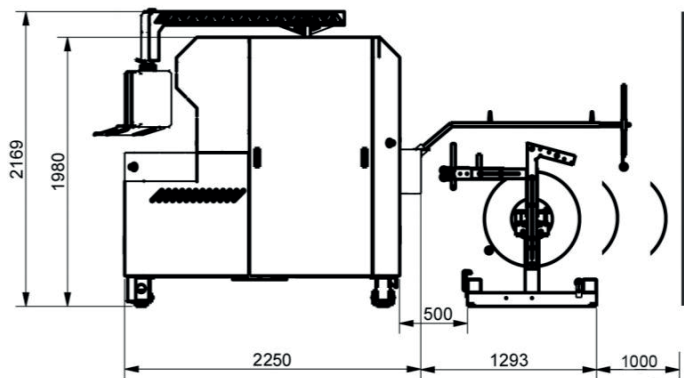
Вид сбоку
