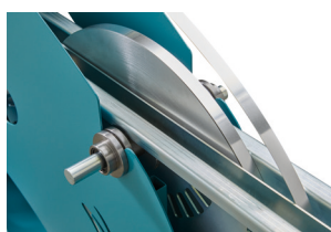
Prise simultanée de deux rouleaux de feuillard
